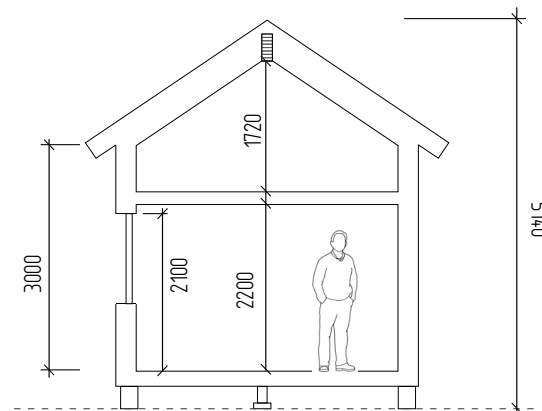
SEKTION A-A
