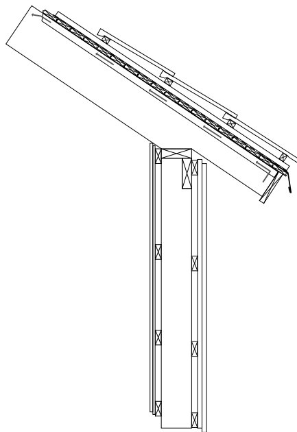
VÄGG/TAK-SNITT
