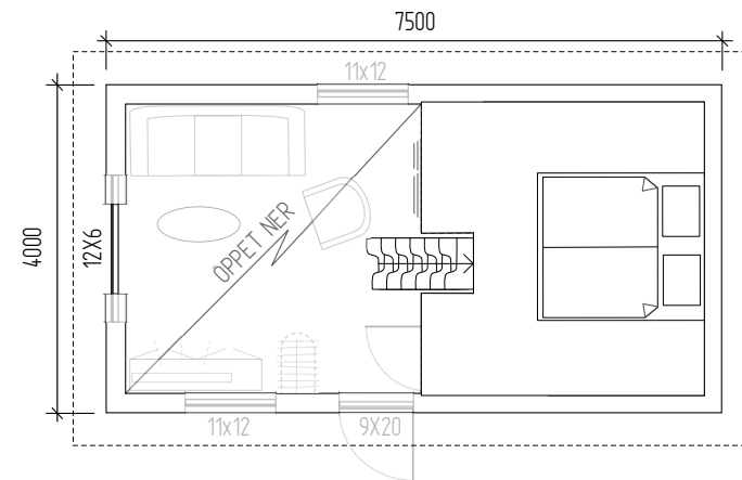
SOVLOFT
